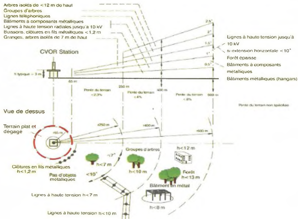
Figure 1 : Surface de protection des signaux du CVOR
