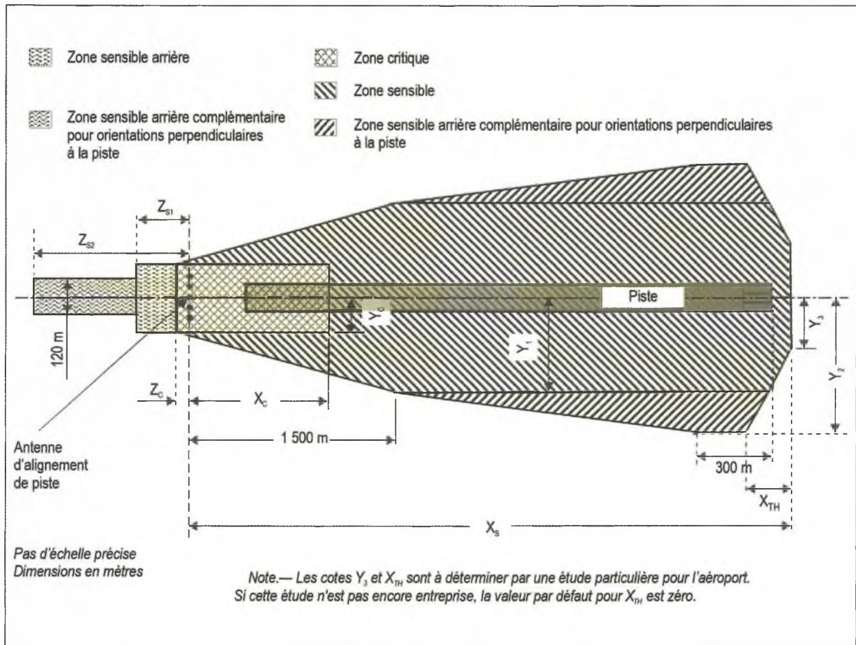
Figure 2. Exemple de dimensionnement de la zone sensible et de la zone critique d'un radiophare d'alignement de piste.
