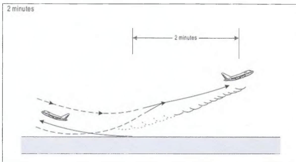
Figure 5-45. Séparation de 2 minutes au titre de la turbulence de sillage, pour des décollages en sens opposé [voir 5.8.5 a)]
