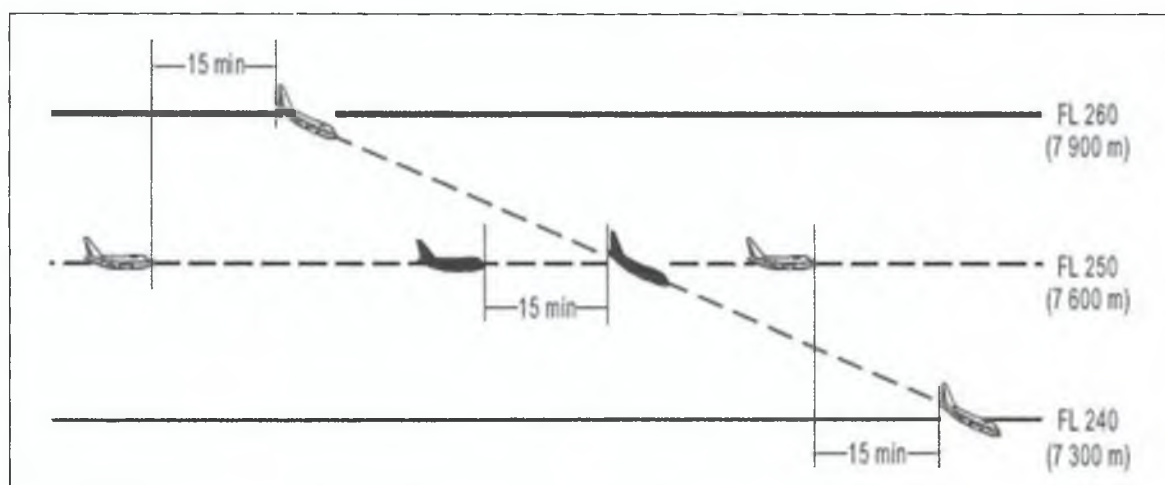
Figure 5-16B. Séparation de 15 minutes entre aéronefs en descente sur la même route [Voir 5.4.2.2.1 a)]
