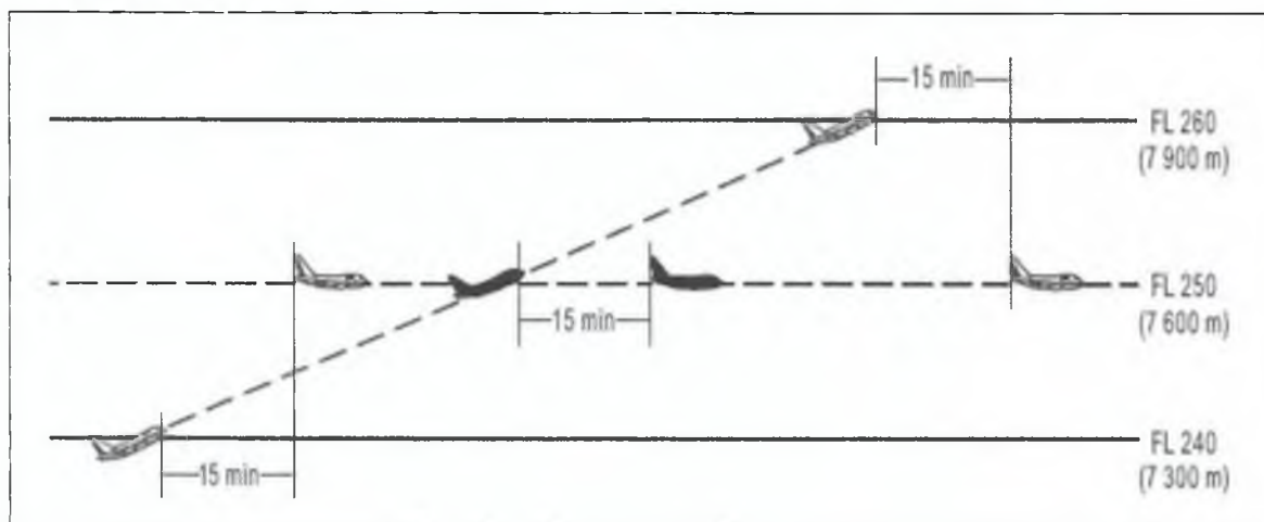
Figure 5-16A. Séparation de 15 minutes entre aéronefs en montée sur la même route [Voir 5.4.2.2.1 a)]
