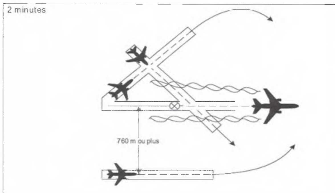
Figure 5-43. Séparation de 2 minutes au titre de la turbulence de sillage, pour l'aéronef qui traverse le sillage [voir 5.8.3.1 c) et d)]
