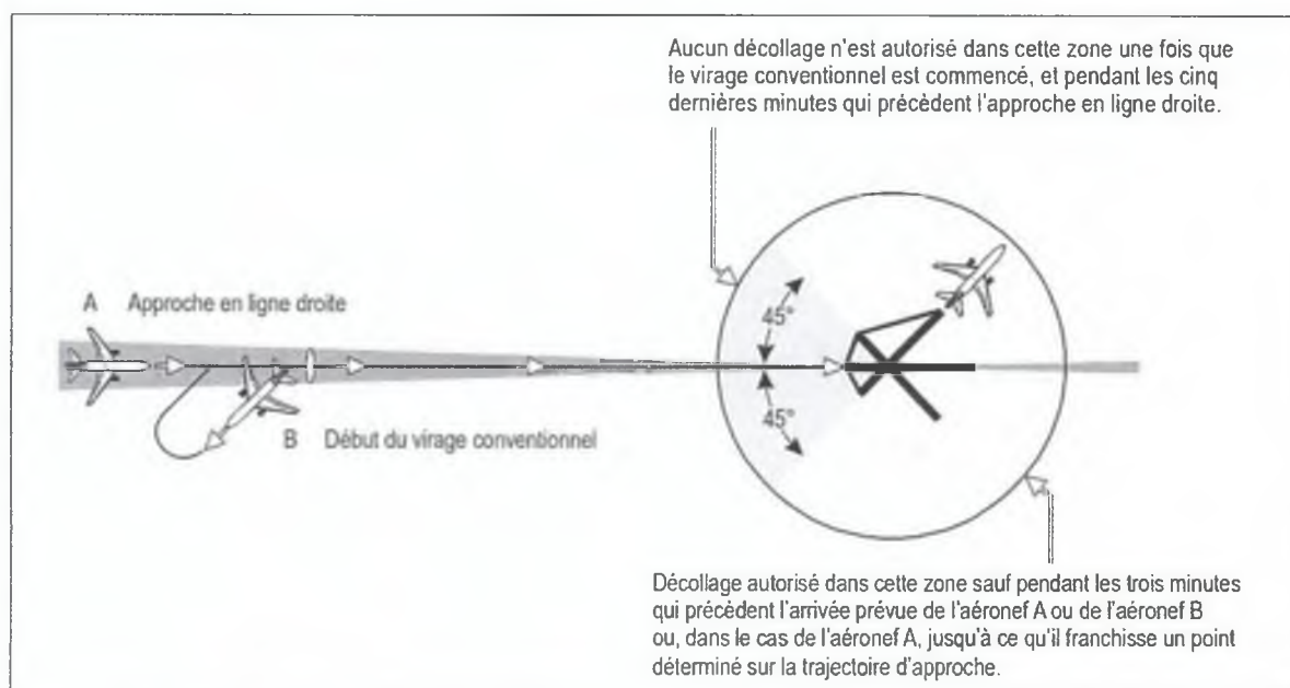
Figure 5-40. Séparation entre aéronefs au départ et aéronefs à l'arrivée [voir 5.7.1.1 b) et 5.7.1.2 b)]
