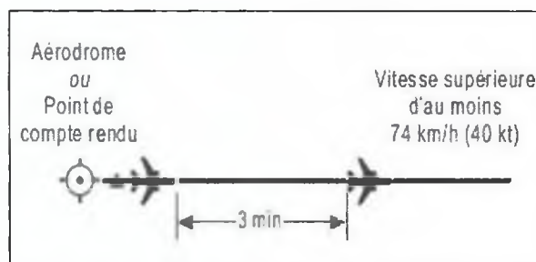
Figure 5-13. Séparation de 3 minutes entre aéronefs sur la même route et au même niveau [Voir 5.4.2.2.1.1 d)]
