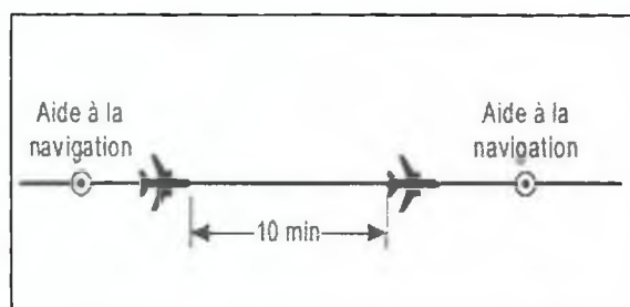
Figure 5-11. Séparation de 10 minutes entre aéronefs sur la même route et au même niveau [Voir 5.4.2.2.1.1 b)]
