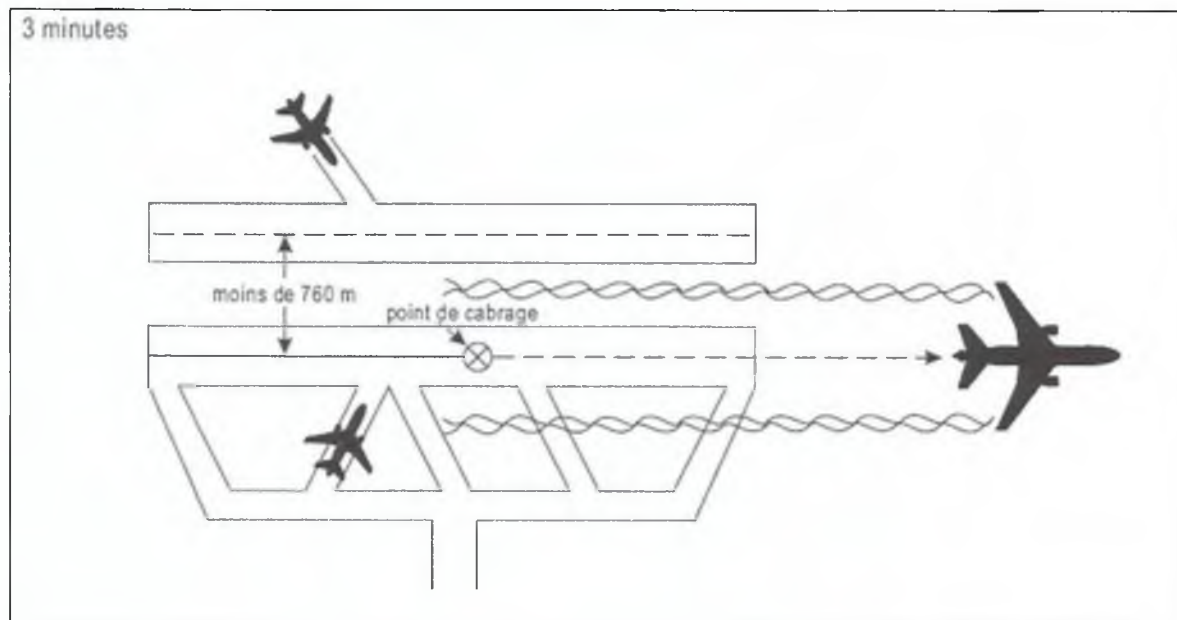
Figure 5-44. Séparation de 3 minutes au titre de la turbulence de sillage, pour l'aéronef qui suit (voir 5.8.3.2)
