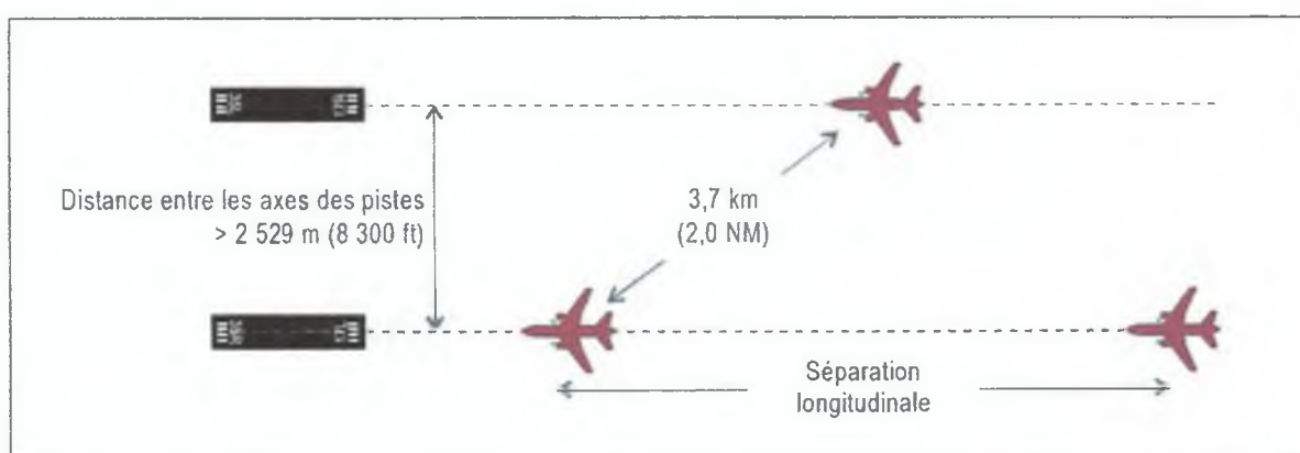
Figure 6-3. Séparation diagonale lorsque la distance entre les axes des pistes
