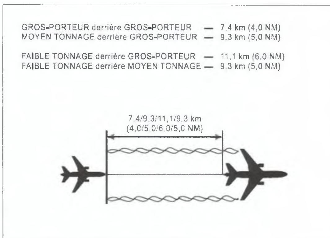
Figure 8-1A. Vol directement dans le sillage (voir 8.7.3.4 et 8.7.4.3.4.1)
