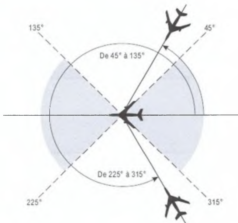
Figure 5-9. Aéronefs sur des routes convergentes [voir 5.4.2.1.5 c)]
