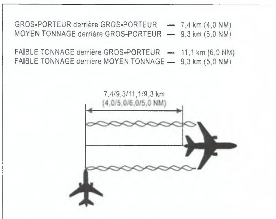
Figure 8-1B. Vol en travers du sillage (voir 8.7.3.4 et 8.7.4.3.4.1)
