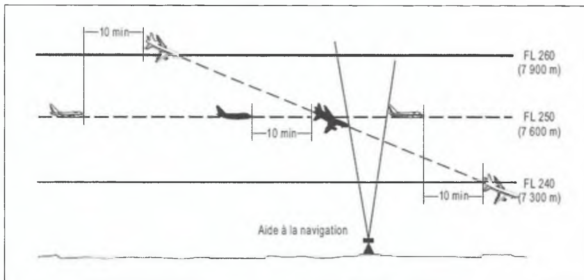
Figure 5-20B Séparation de 10 minutes entre aéronefs en descente sur des routes convergentes [Voir 5.4.2.2.2.2 b)]
