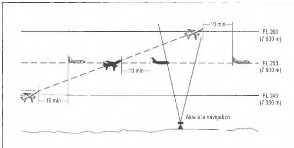
Figure 5-20A. Séparation de 10 minutes entre aéronefs en montée sur des routes convergentes [Voir 5.4.2.2.2.2 b)]
