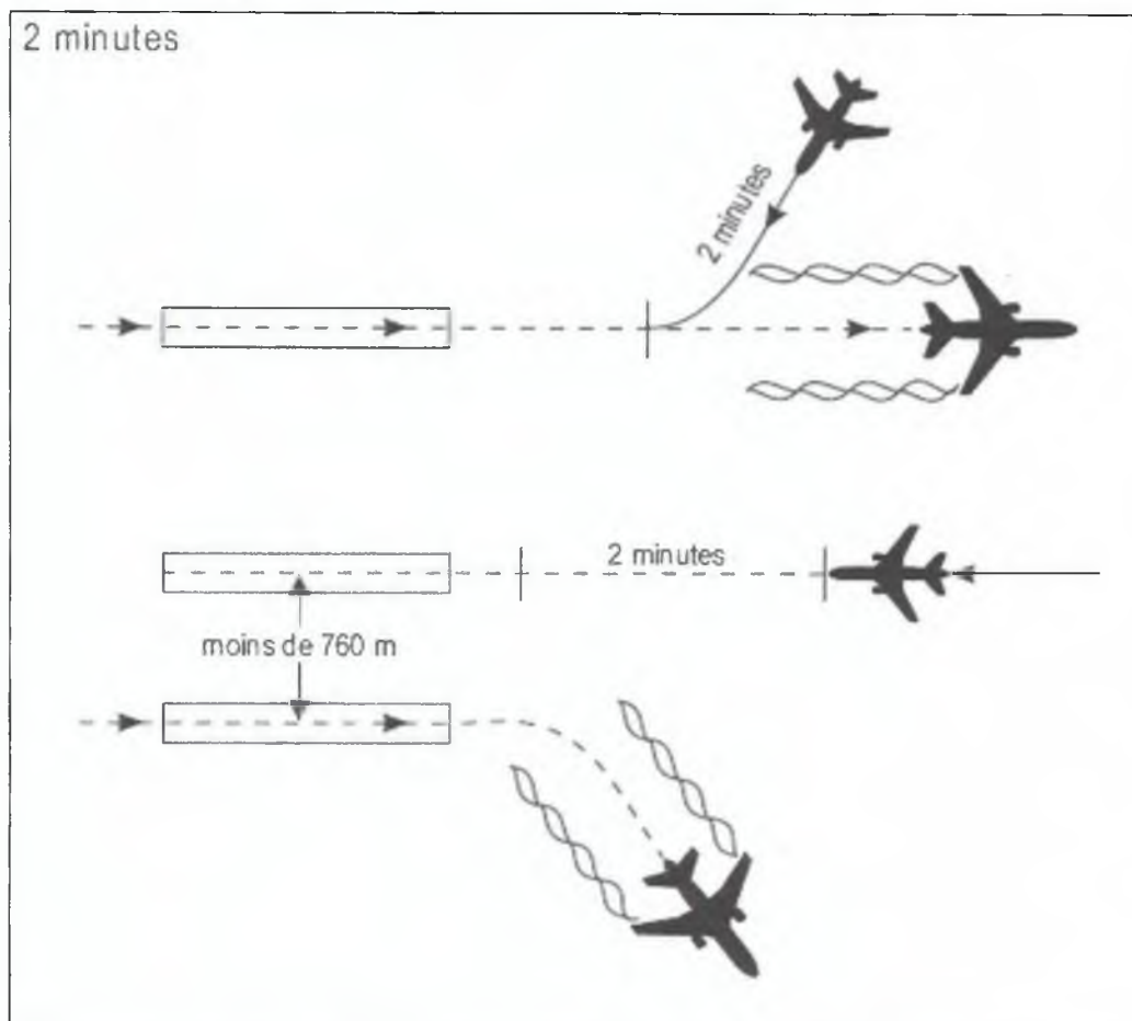
Figure 5-46. Séparation de 2 minutes au titre de la turbulence de sillage, Pour des atterrissages en sens opposé [voir 5.8.5 b)]
