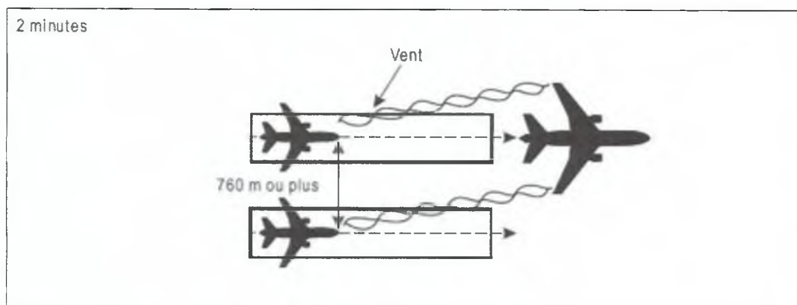
Figure 5-42. Séparation de 2 minutes pour l'aéronef qui suit [voir 5.8.3.1 a) et b)]
