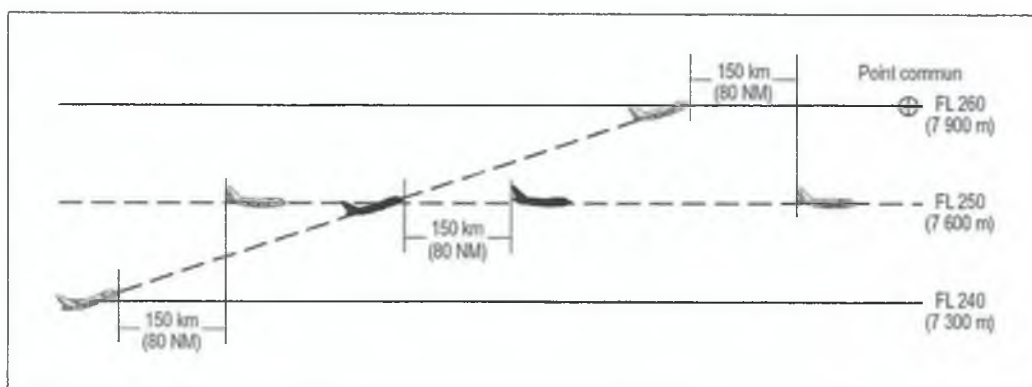
Figure 5-27A. Séparation fondée sur une distance RNAV de 150 km (80 NM) entre aéronefs en montée sur la même route [voir § 5.4.2.5.5, c)]
