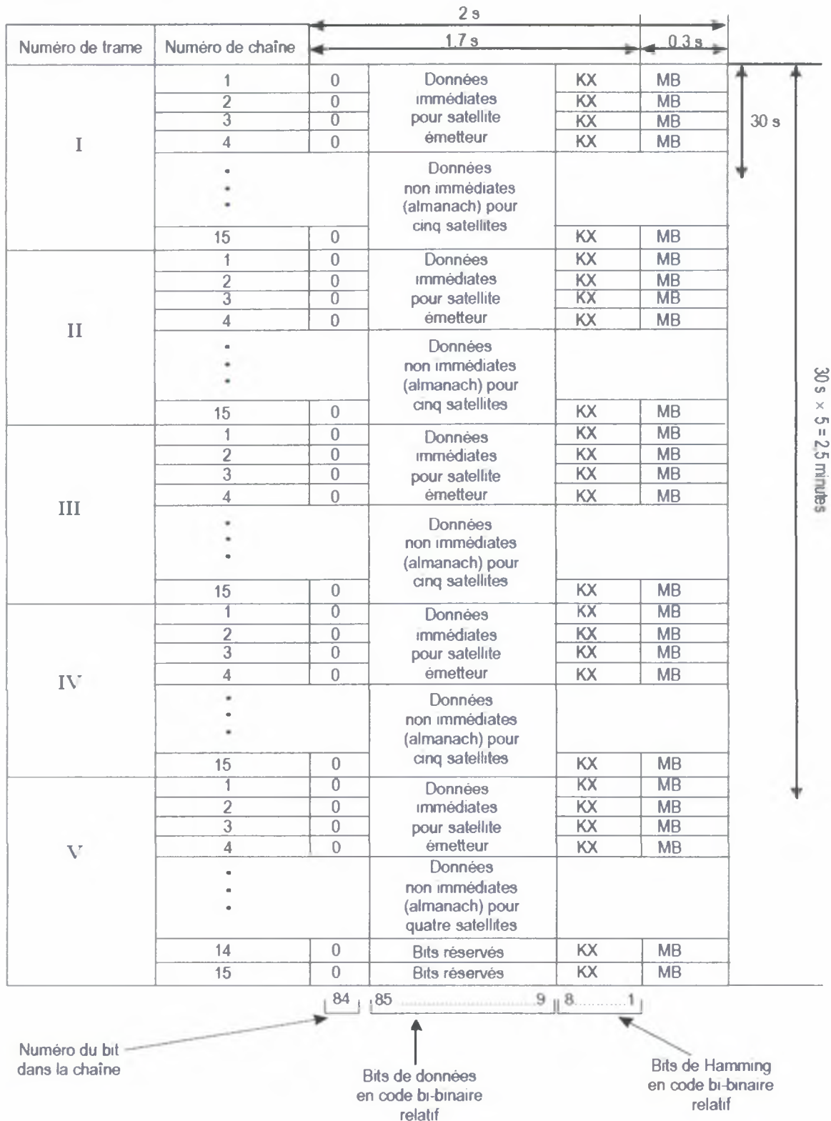
Figure B-7. Structure de la supertrame
