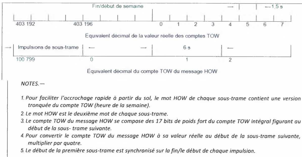
Figure B-5. Schéma temporel du HOW
