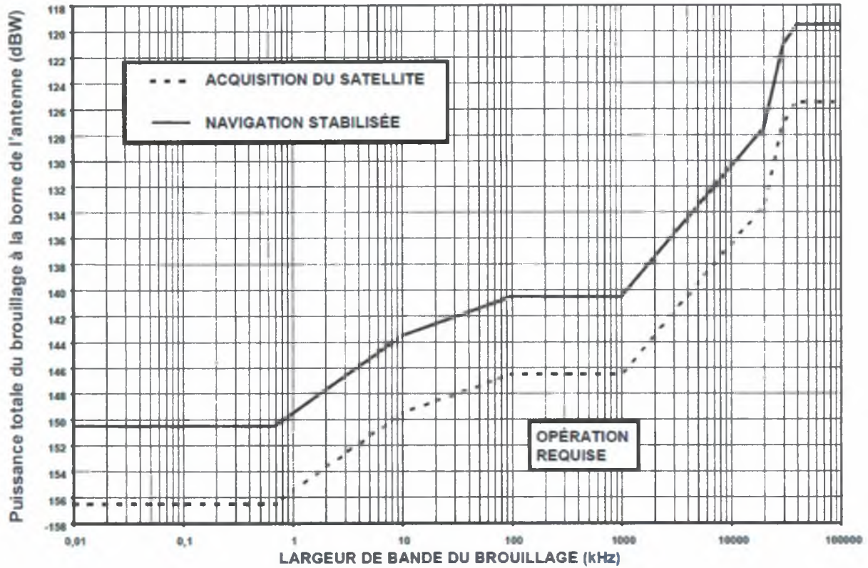
Figure B-17. Seuil de brouillage en fonction de la largeur de bande (récepteurs GPS et SBAS)
