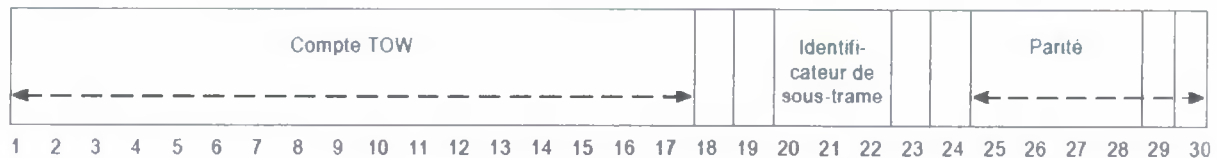
Figure B-4. Format du mot HOW
