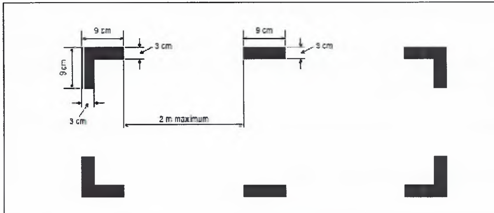
INDICATION DES ZONES DE PÉNÉTRATION DU FUSELAGE (voir § 2.4.2.6)
